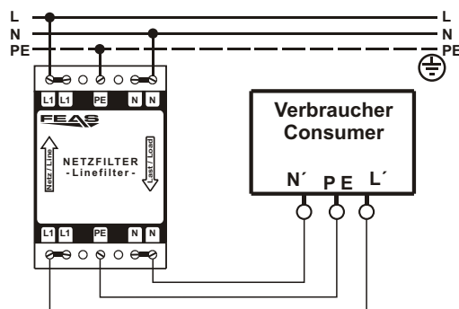
Anschlußbeispiel
