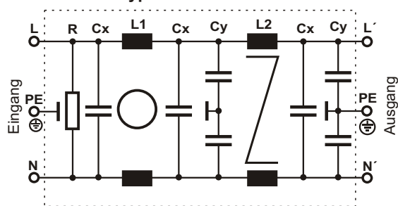
Typisches Schaltbild
