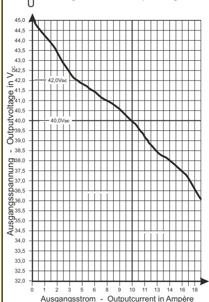
U - I Verlauf bei 230V Eingangsspannung U - I Diagram with 230V Inputvoltage
