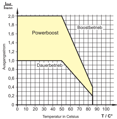
Laststromdiagramm bei nominaler Eingangsspannung
