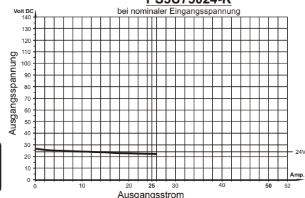
Laststromdiagramm PS3U75024-K bei nominaler Eingangsspannung
