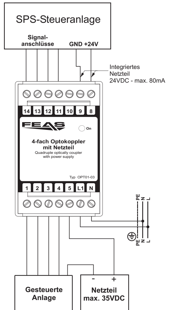
Anschlußbeispiel
