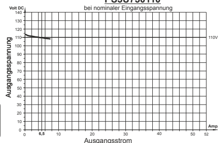
Laststromdiagramm PS3U750110 bei nominaler Eingangsspannung
